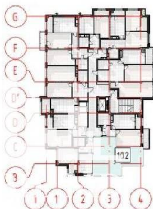
Borderoul incaperi (P+1E, cota 2.900) apartament "102" - 1 odaie, cu nr. cad. 0100201.197.03.011
