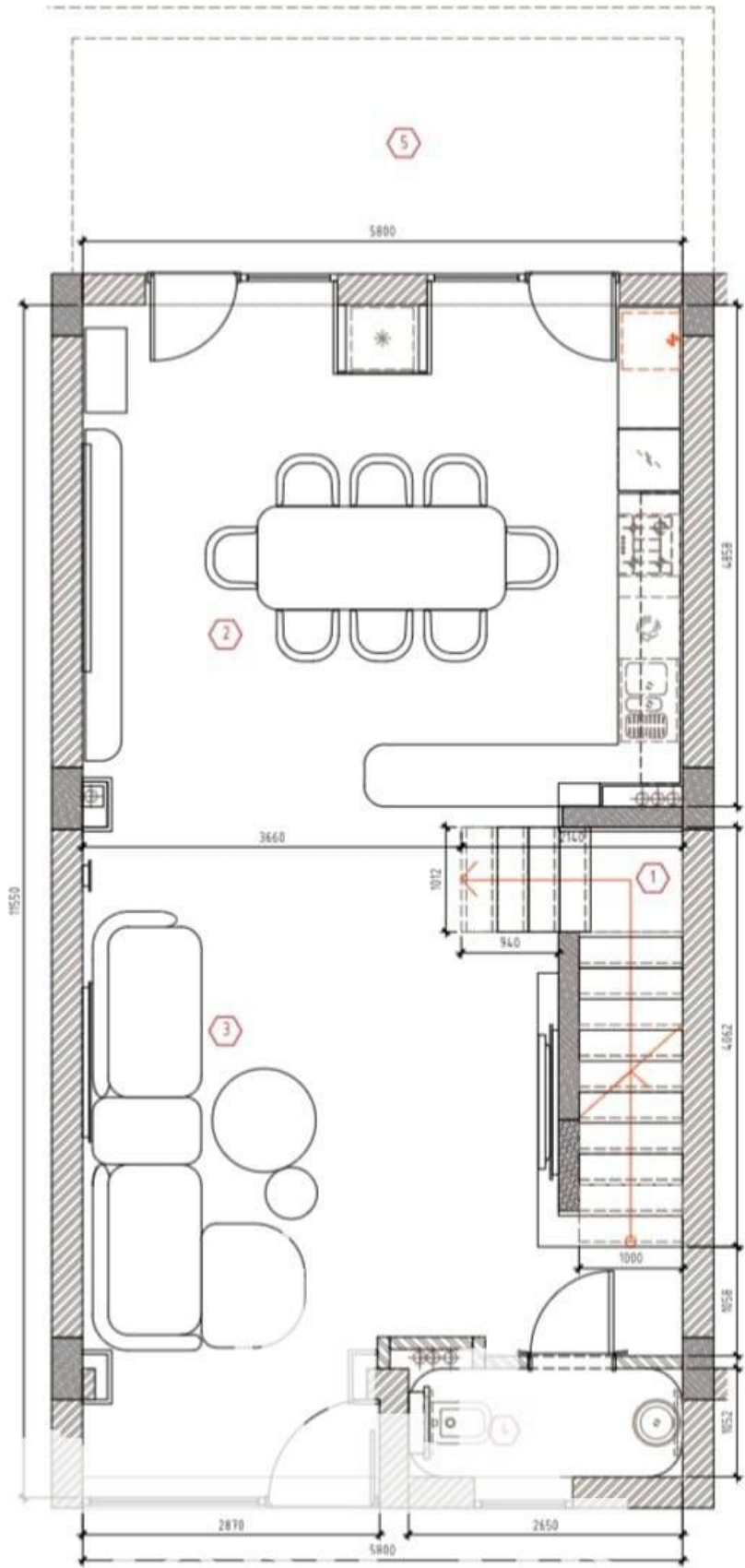
План (1 этаж отн. 0.000)
