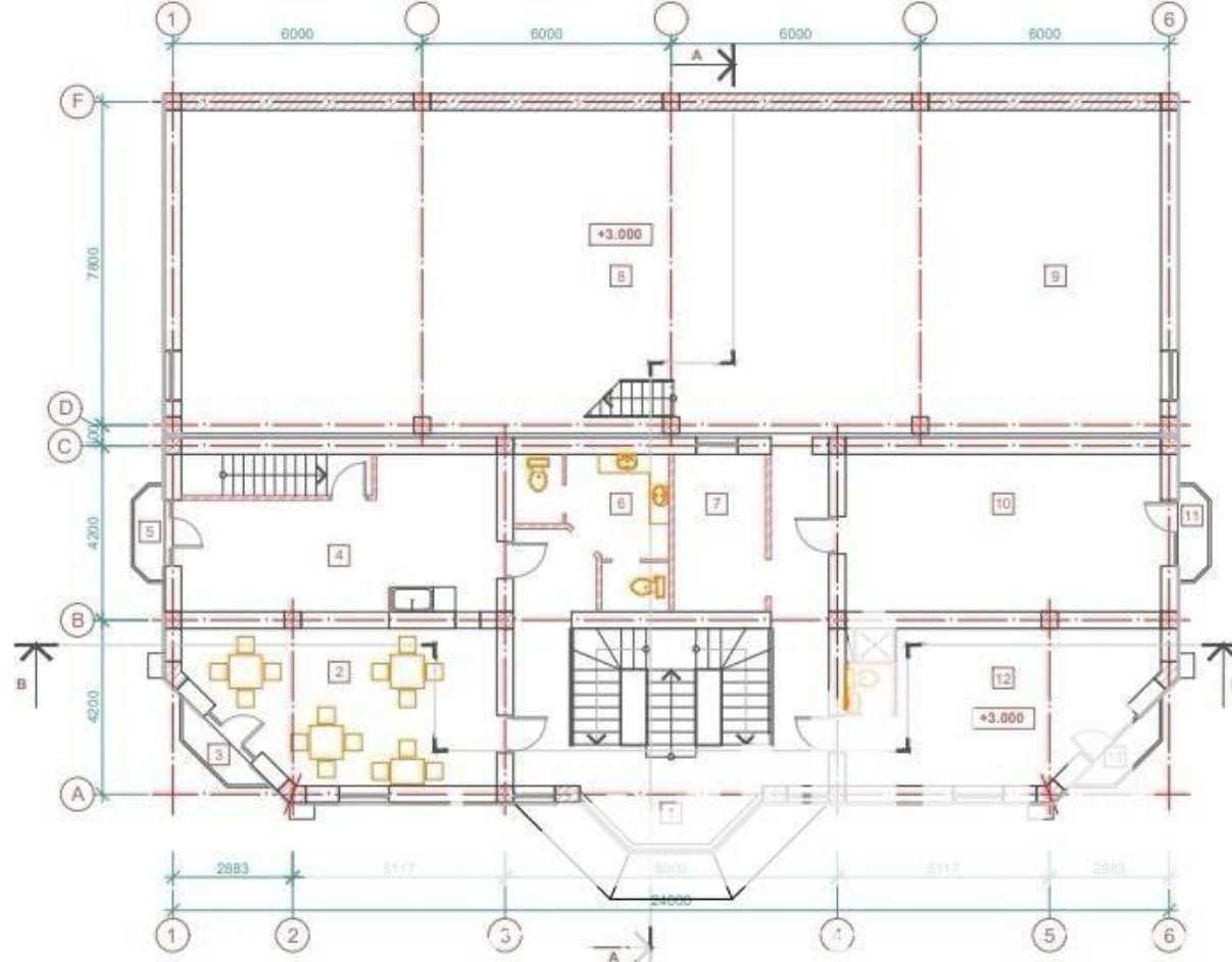
LEGENDA INCAPERILOR
