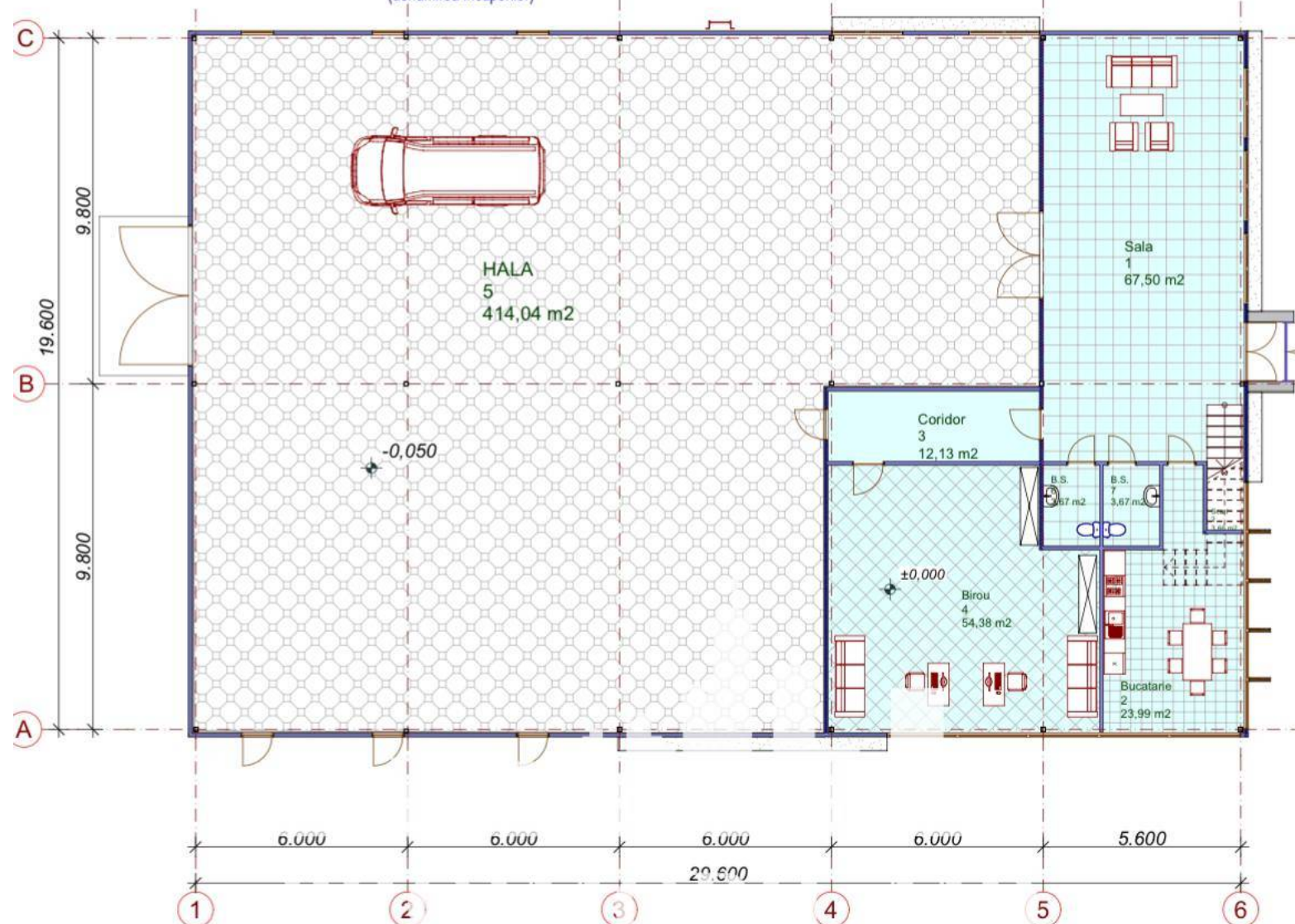
PLAN PARTER, cota 0.000 Sc. 1:100 (denumirea incaperilor)
