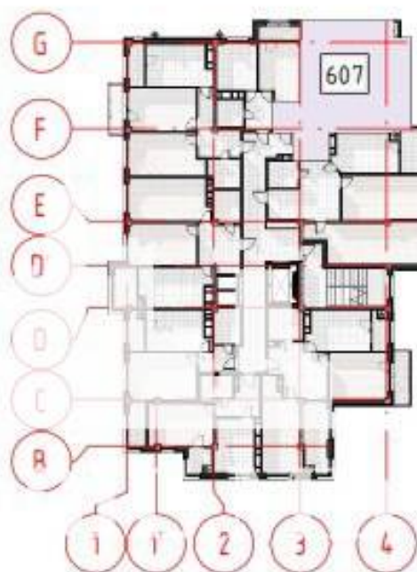
Borderoul incaperi (P+6E, cota 17.400) apartament "607" - 2 odai, cu nr. cad. 0100201.197.03.059
