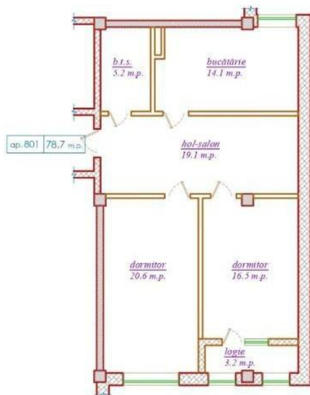
schema amplasare ap. nr. 801
