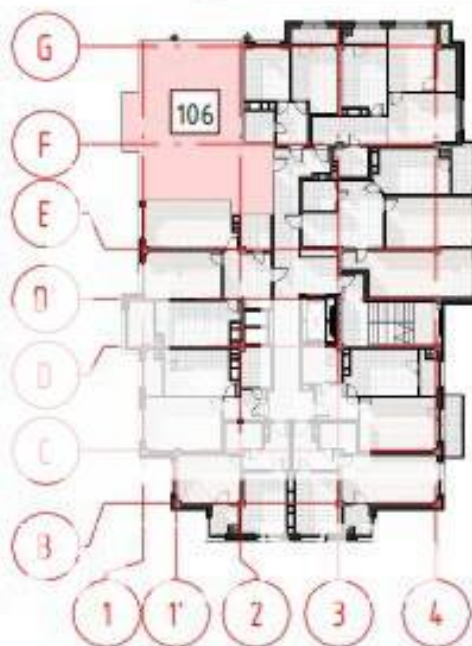
Borderoul incaperi (P+1E, cota 2.900) apartament "106" - 2 odai, cu nr. cad. 0100201.197.03.015
